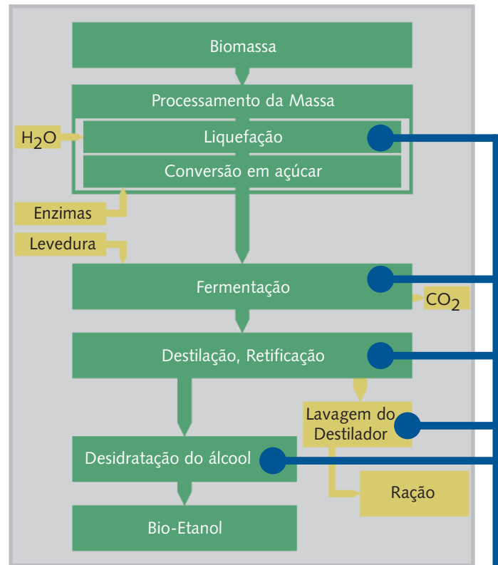
Processo de produção do Bio-Etanol - Fermentação
